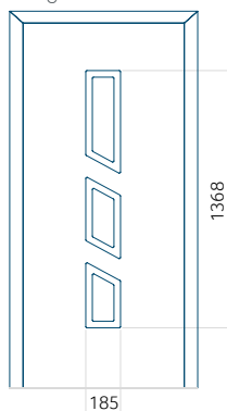
Disegno tecnico
