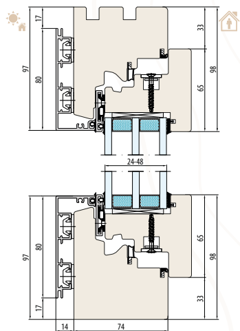
SISTEMA ESPERIA LIFE 74 ALU Senza scanalatura per il davanzale
