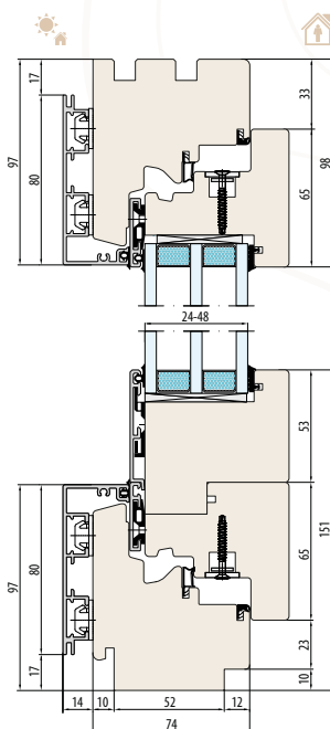
SISTEMA ESPERIA LIFE 74 ALU Porte balcone a una anta con soglia alta
