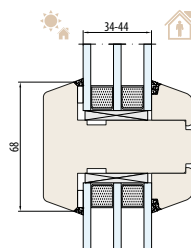
SISTEMA NATURO 80 Montante strutturale 68 mm
