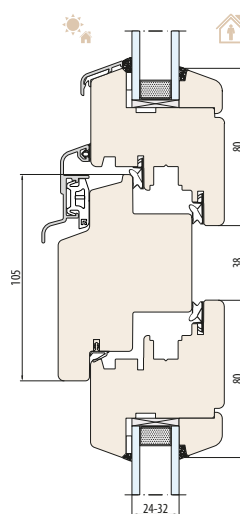
SISTEMA NATURO 68 Traverso 105 mm
