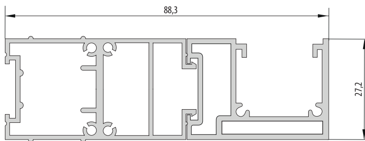
Guida monoblocco SOLID
