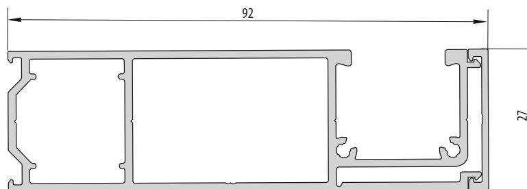
Guida monoblocco Eko-Okna
