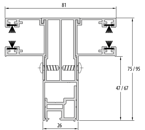
• Guida di divisione RGT 75/95 • Roka top 2 RG / RG EX
