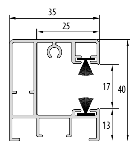
• PPA 35/17* • Opoterm, Styrotherm
