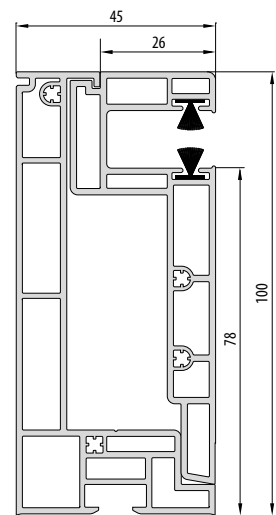
• PPRA 12** • Styroterm con ispezione dall'esterno
