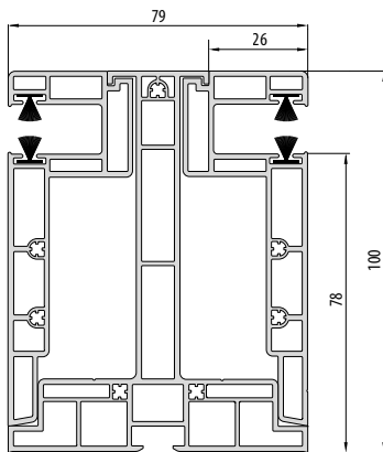
• PPDR 79 • Styroterm con ispezione dall'esterno
